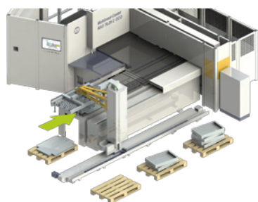
Séparation et chargement d'une plaque avec le système de chargement RAS Palletizer
