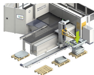
Empilement horizontal d'une pièce pliée sur une palette
