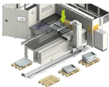
Prise de la pièce pliée par le cadre d'aspiration du Palletizer
