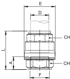
raccord droit femelle
