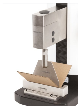
Test de pliage d'emballage
