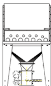
Avec microdoseur MBF
