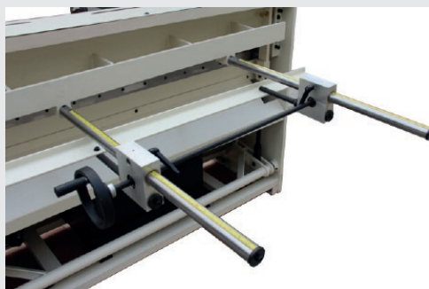
FIG.: OPTION BUTÉE ARRIÈRE (RÉGLABLE PAR VOLANT)
