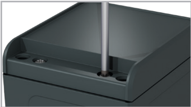
Visser le couvercle avec seulement deux vis après avoir accroché les pivots.
