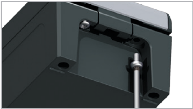
Bloquer le pivot de la charnière avec 2 vis.
