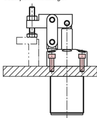
Par le haut avec quatre vis CHC à travers la bride.
