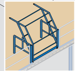
Barrière écluse
