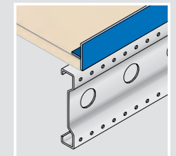
Panneau aggloméré avec protection d'angle, superposé
