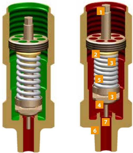
Fermée Ouverte
