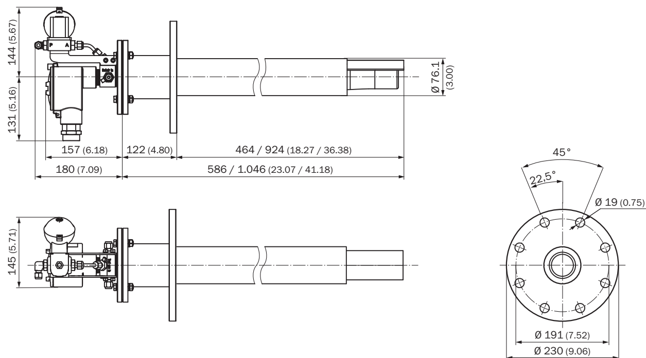
Analyseur ZIRKOR200 Ex-G
