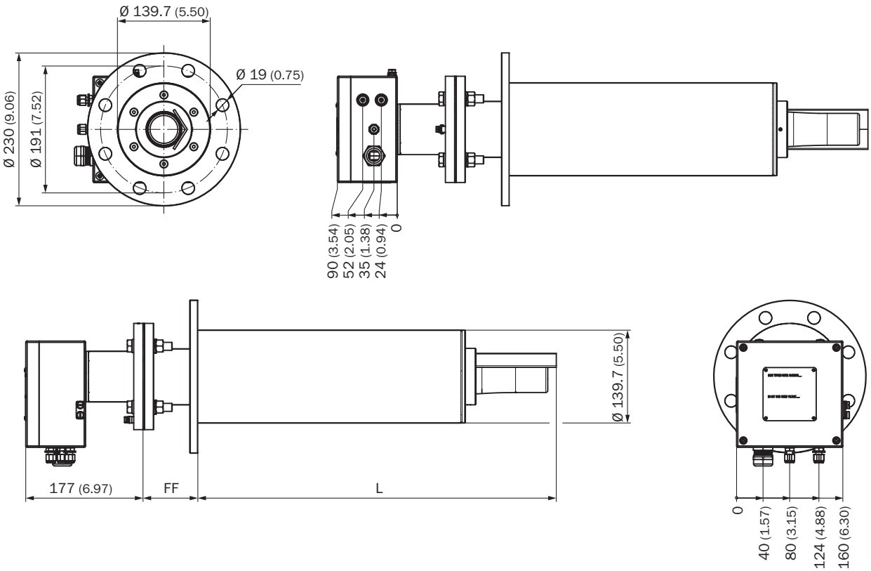
Analyseur ZIRKOR200 Ex-D
