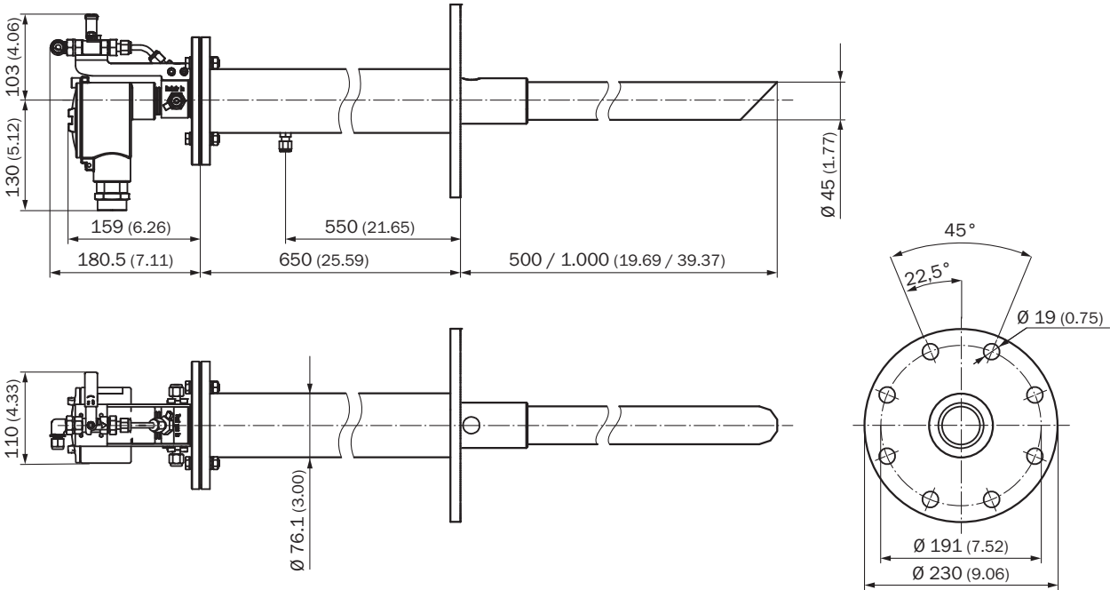
Analyseur ZIRKOR200 Ex-G avec vanne manuelle et tube de protection antigel
