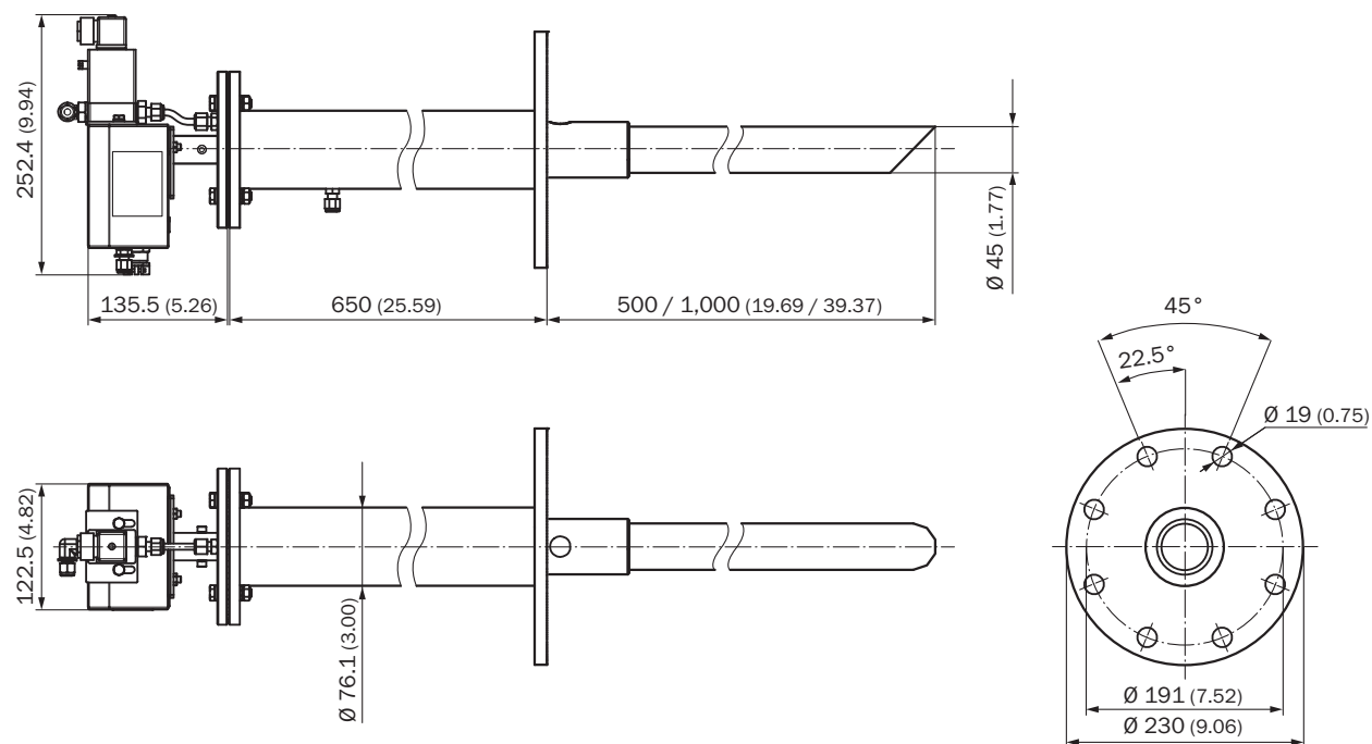
Analyseur ZIRKOR200 avec tube de protection antigel
